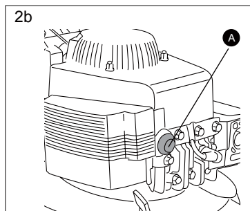
2b Press the primer bulb (A) 3-5 times.
